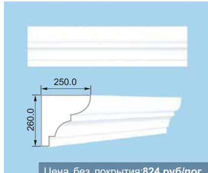
Подоконник 5
