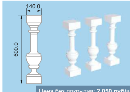
Балясина 2
