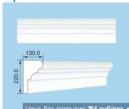
Карниз 17
