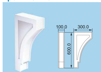
Кронштейн 3
