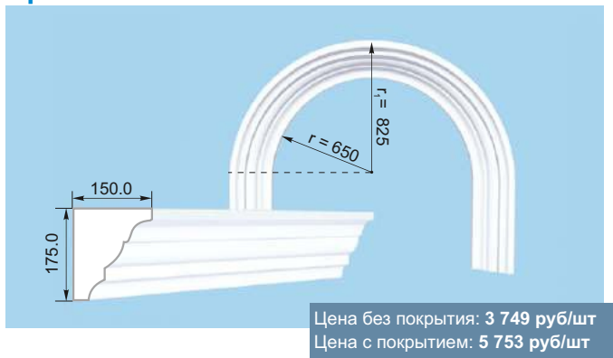
Арка 05
