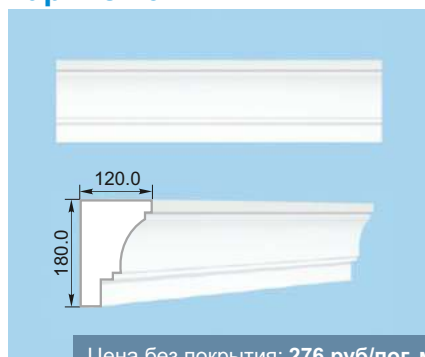
Карниз 23
