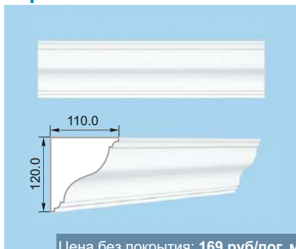
Карниз 31
