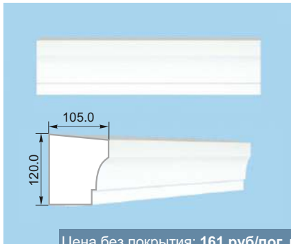
Подоконник 7
