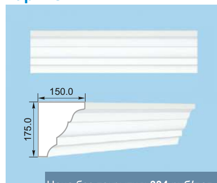
Карниз 24
