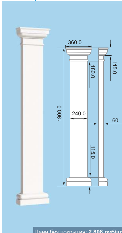
Пилястра 1
