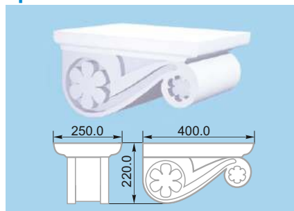
Кронштейн 5
