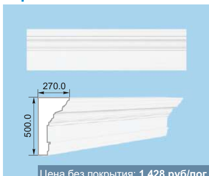
Карниз 34
