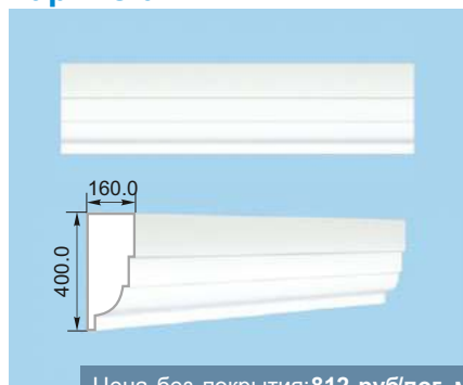
Карниз 04
