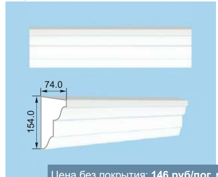
Карниз 27
