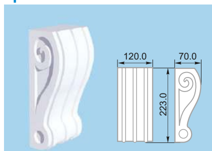
Кронштейн 2
