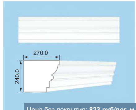
Подоконник 9
