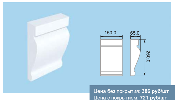
Замковый камень 8
