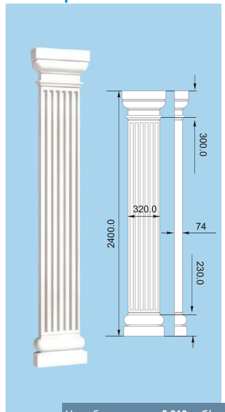
Пилястра 2
