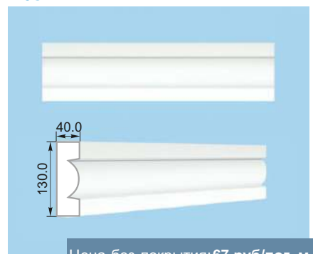
Наличник 12
