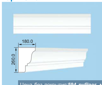
Карниз 16
