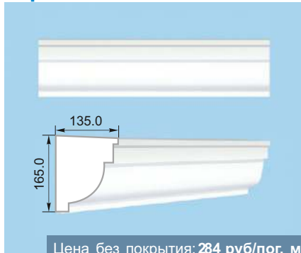
Карниз 25
