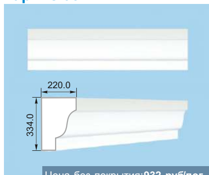
Карниз 05
