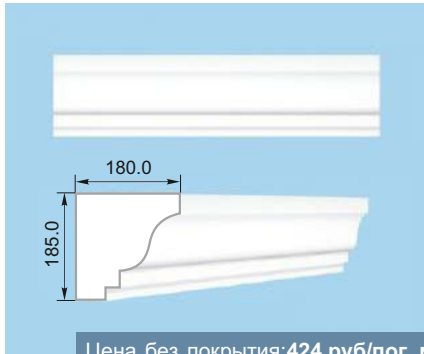
Подоконник 4
