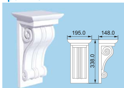
Кронштейн 1
