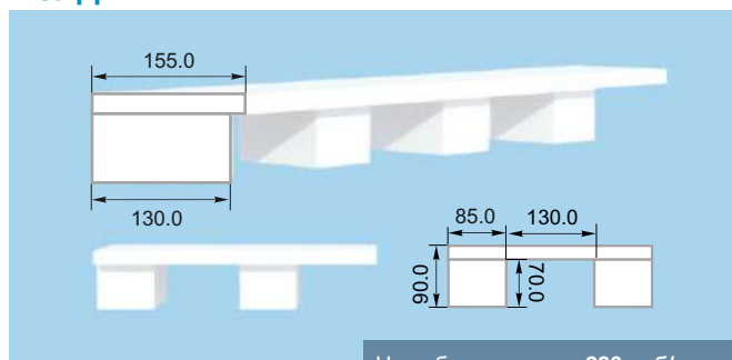
Молдинг 1
