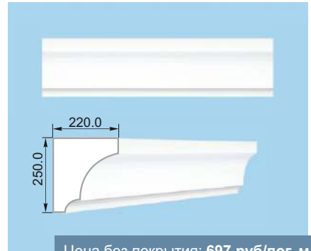
Подоконник 6
