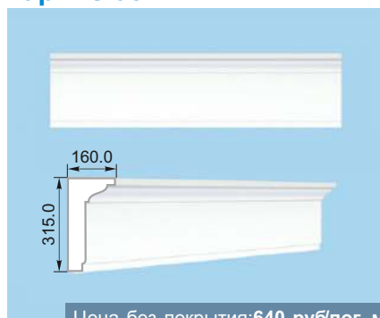
Карниз 08
