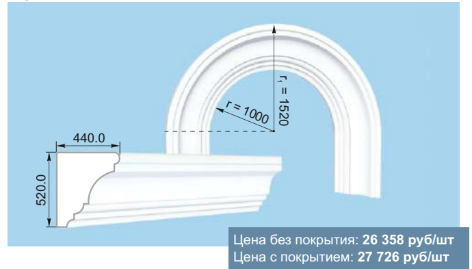
Арка 04
