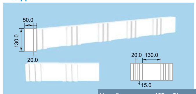
Молдинг 2
