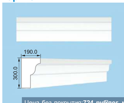
Карниз 11
