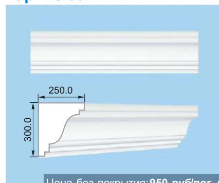
Карниз 09
