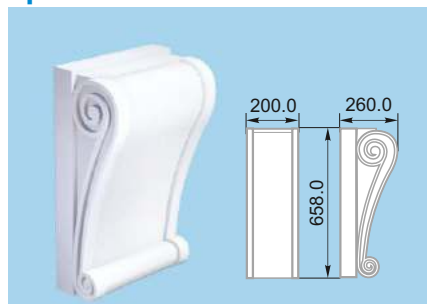
Кронштейн 4
